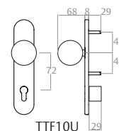
Pull knob
