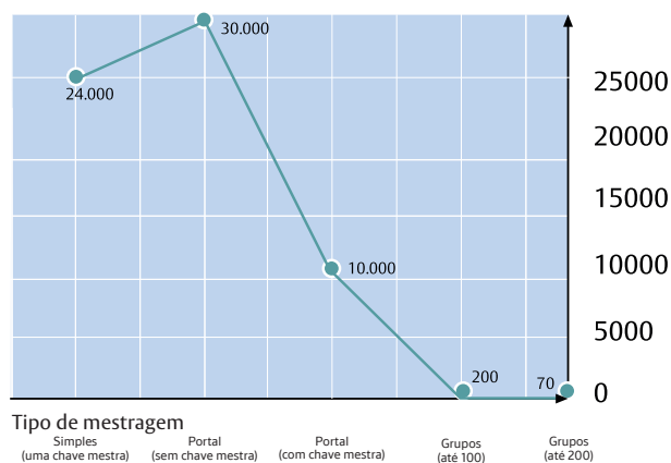
Plataforma PIN TUMBLER + pinos passivos N.º de chaves próprias
